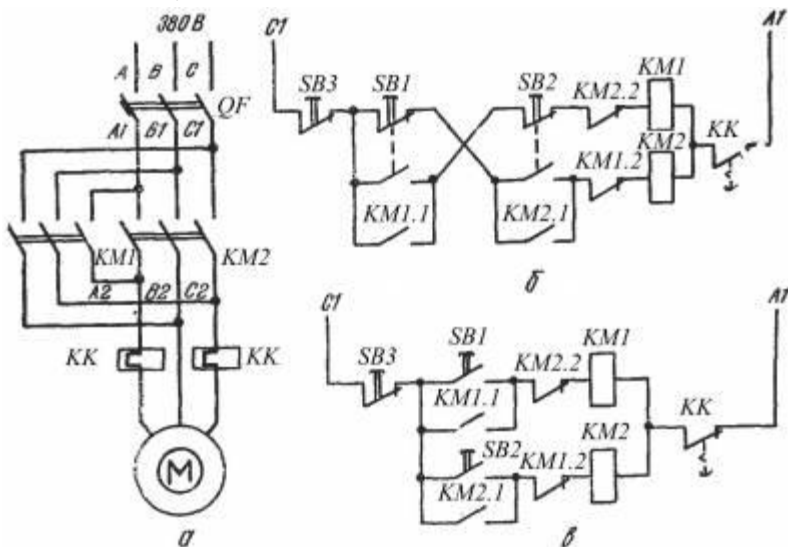
Рисунок 2 – Схема управления электродвигателем с двух мест при наличии соответствующего количества кнопочных станций.
