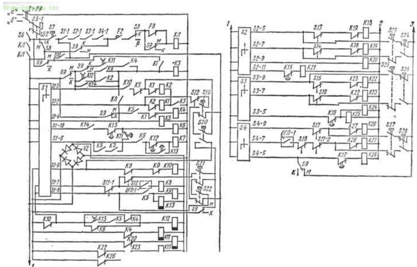
Принципиальная электрическая схема
