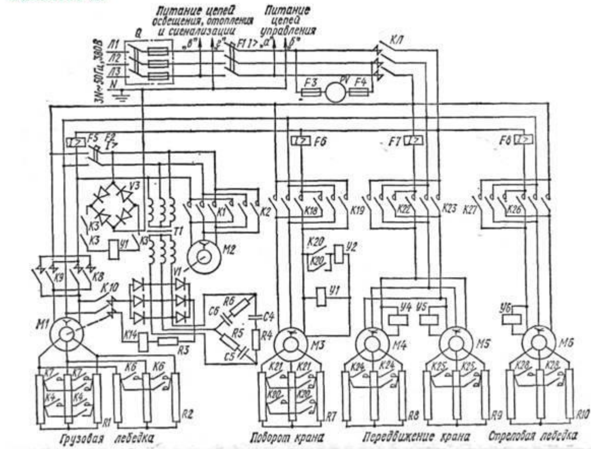
Принципиальная электрическая схема
